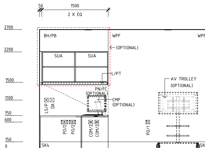
ELEVATION 2
