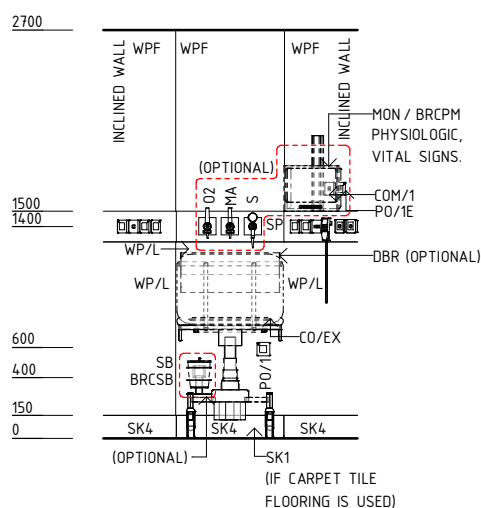
ELEVATION 5
