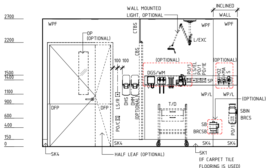
ELEVATION 3
