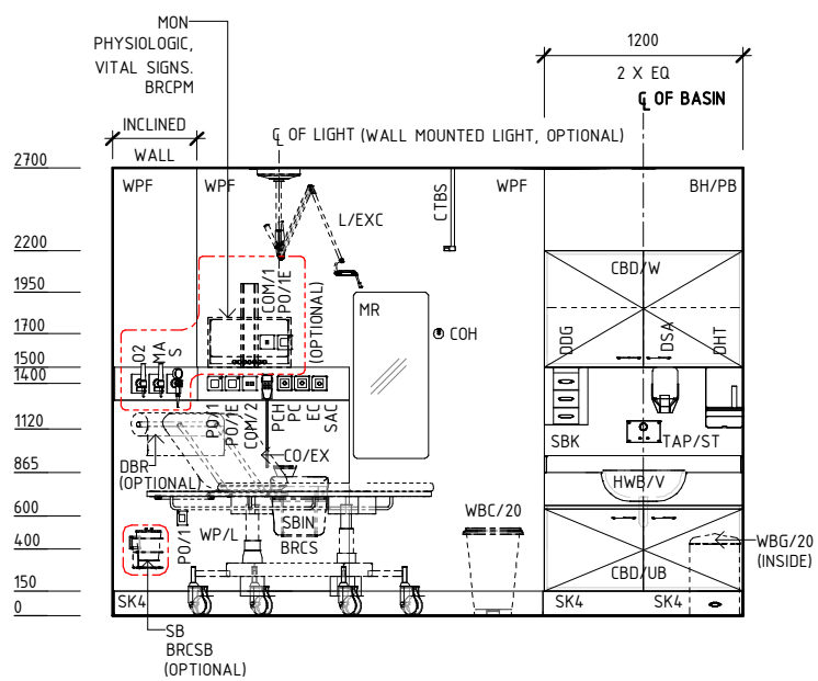
ELEVATION 4
