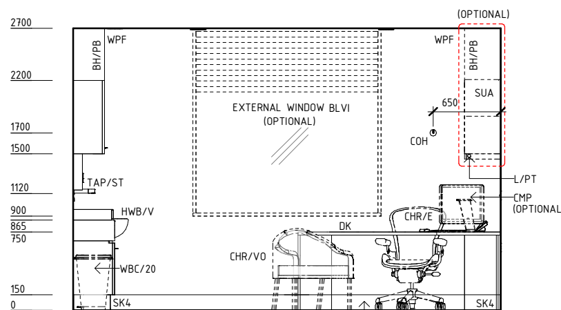
ELEVATION 1
