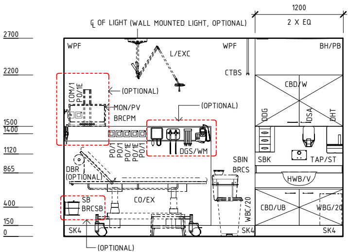
ELEVATION 4
