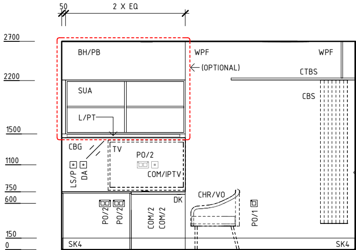
ELEVATION 2
