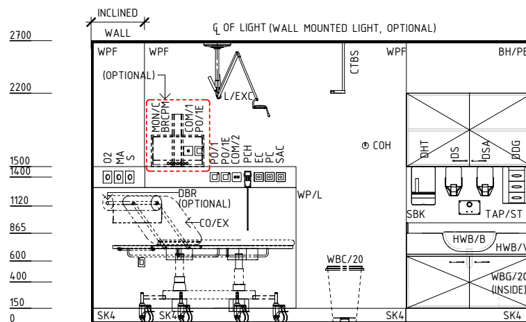
ELEVATION 4
