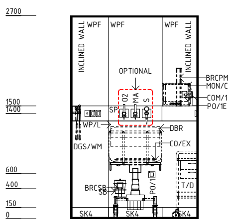
ELEVATION 5
