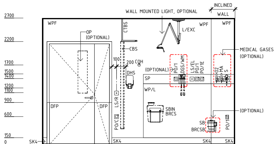
ELEVATION 3
