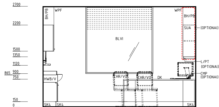
ELEVATION 1
