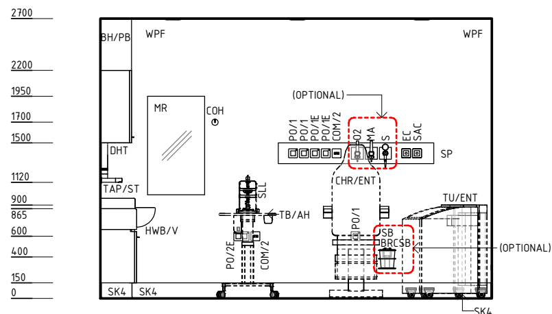
ELEVATION 2
