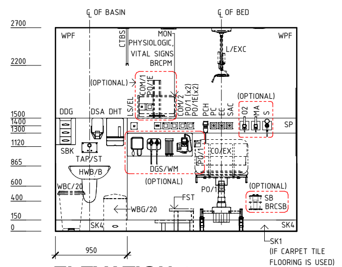
ELEVATION 4
