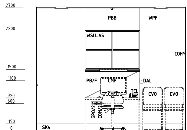
ELEVATION 2
