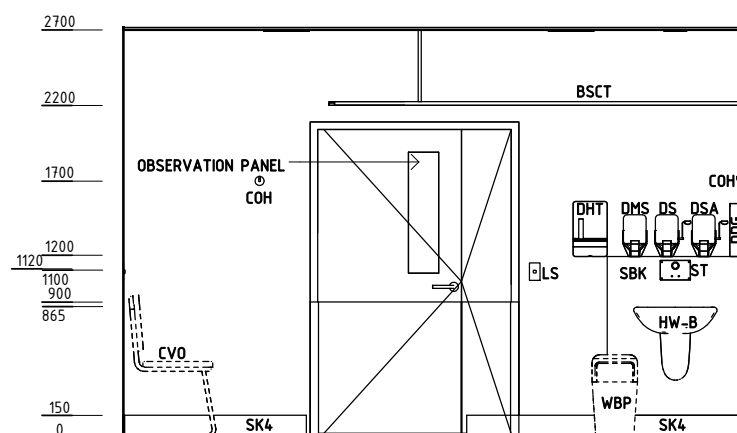
ELEVATION 3
