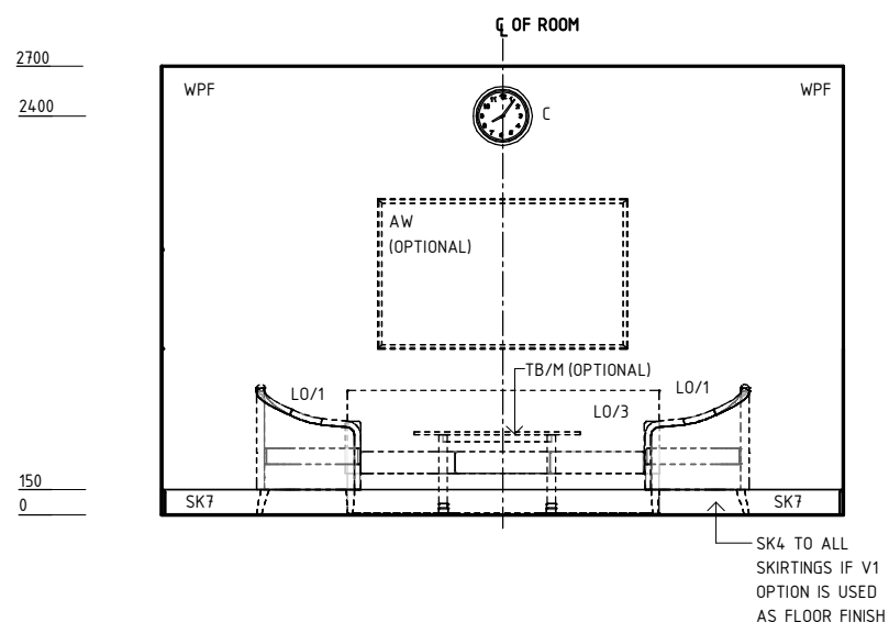
ELEVATION 1
