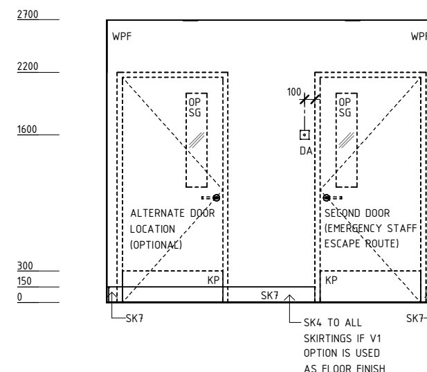
ELEVATION 4
