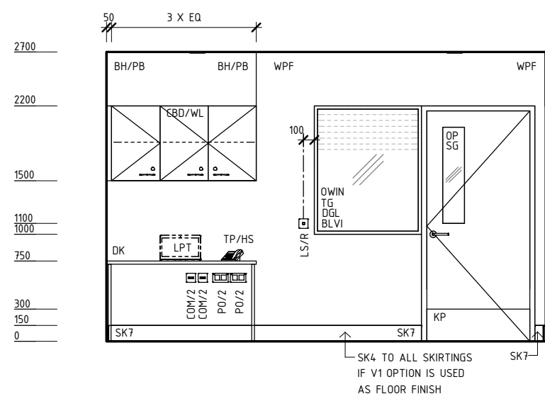
ELEVATION 3
