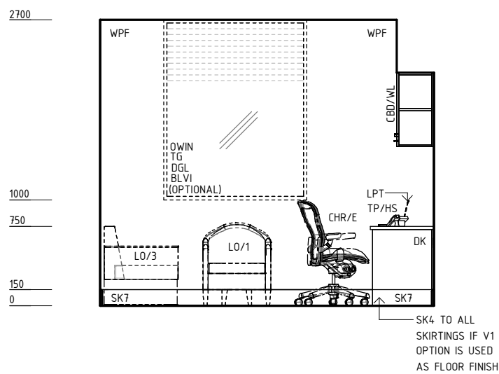
ELEVATION 2
