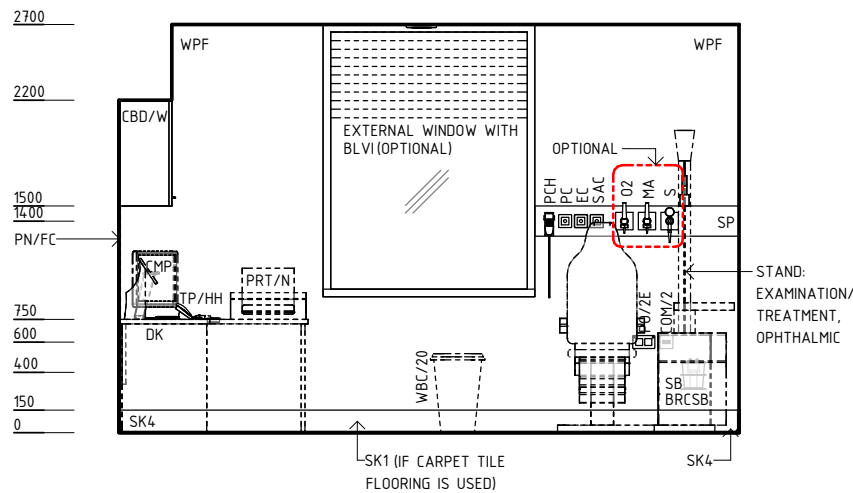
ELEVATION 1
