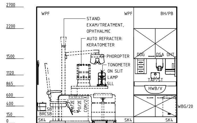
ELEVATION 2
