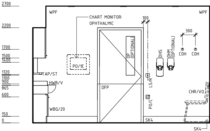
ELEVATION 3
