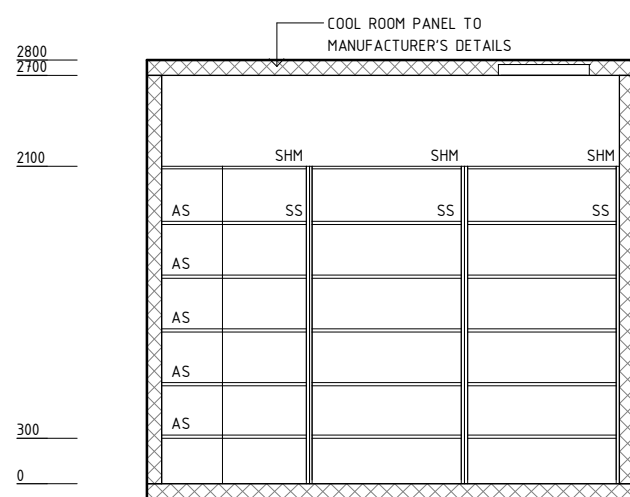
ELEVATION 2
