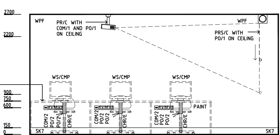
ELEVATION 4
