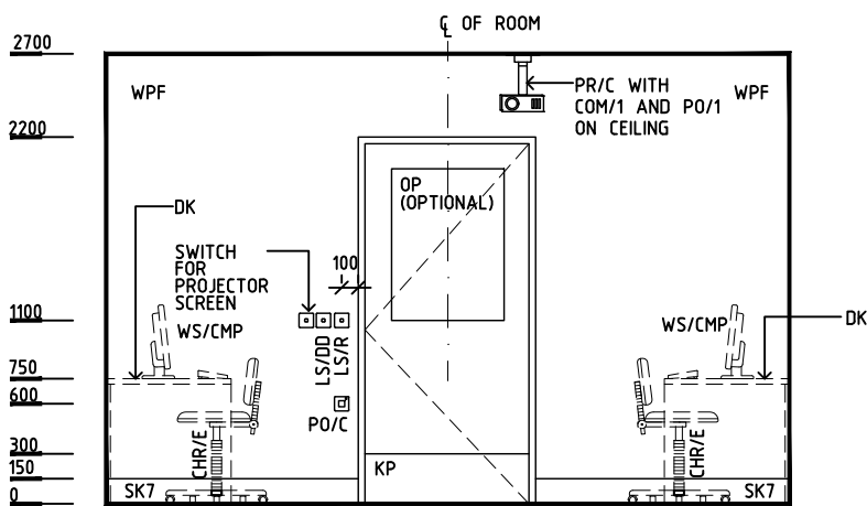
ELEVATION 3
