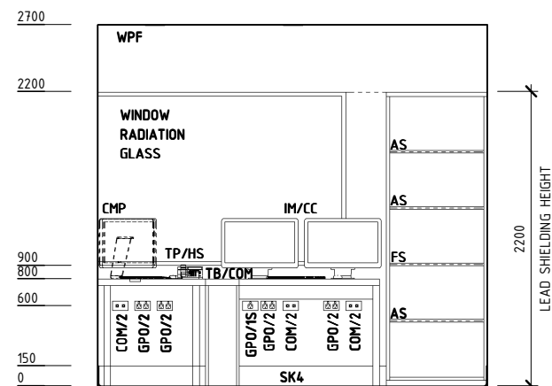
ELEVATION 2
