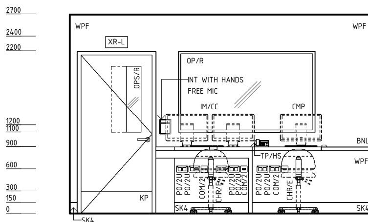
ELEVATION 2
