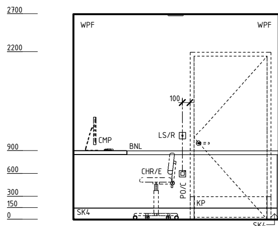
ELEVATION 3
