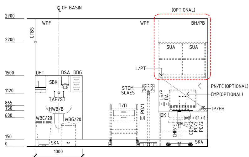
ELEVATION 4
