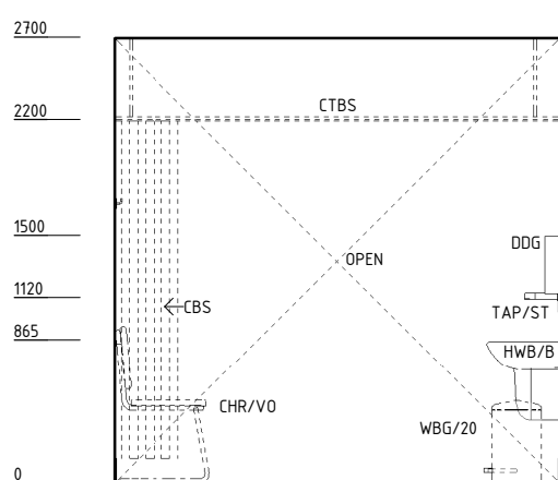
ELEVATION 3
