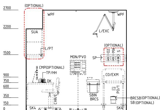
ELEVATION 1
