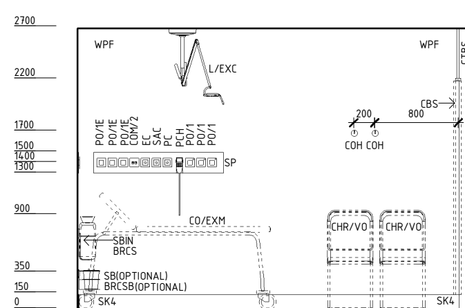
ELEVATION 2
