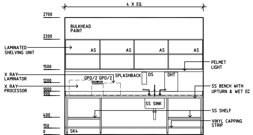
ELEVATION 2
