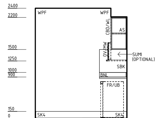
ELEVATION 6
