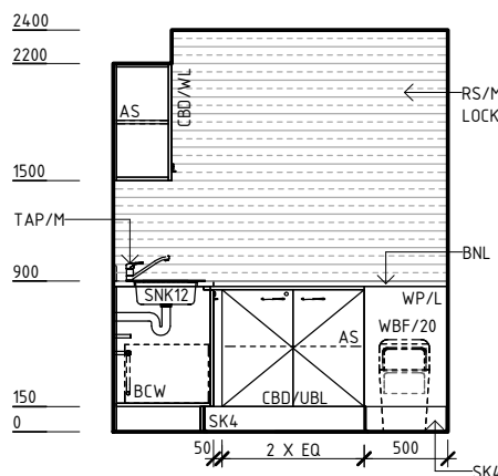
ELEVATION 5
