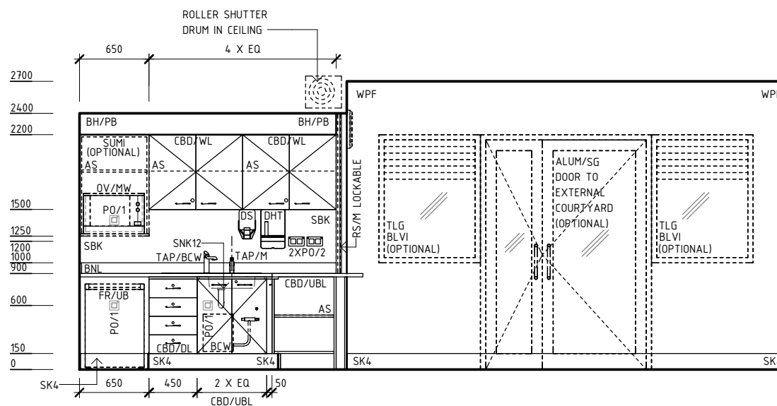
ELEVATION 1
