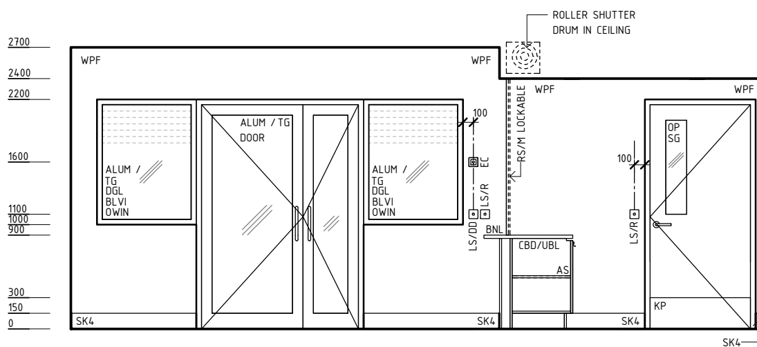
ELEVATION 3
