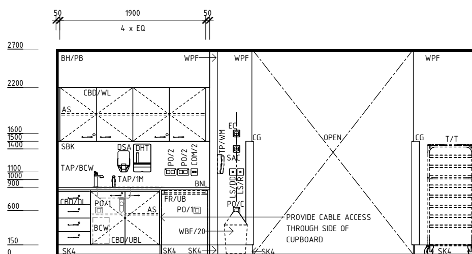
ELEVATION 3
