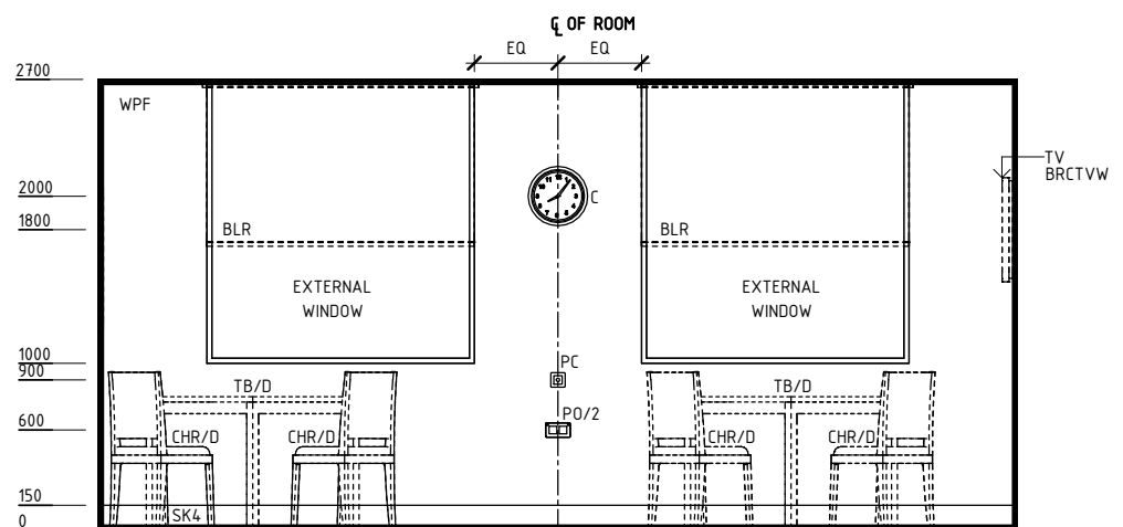
ELEVATION 1
