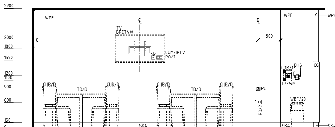
ELEVATION 2
