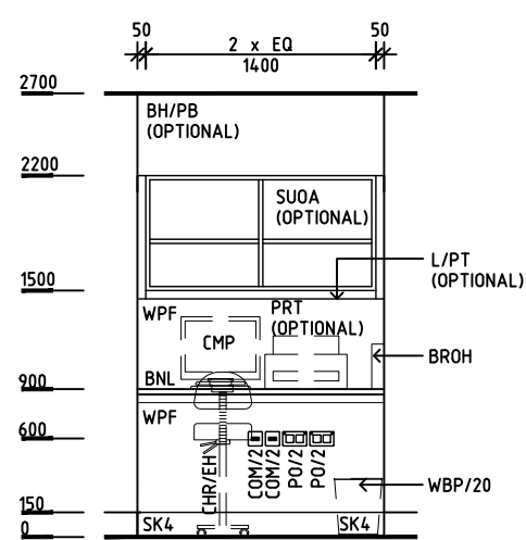
ELEVATION 2
