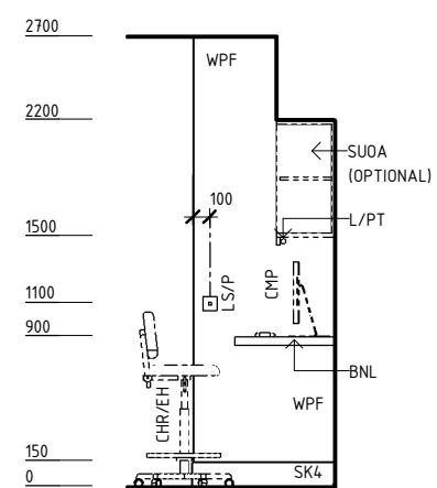
ELEVATION 2
