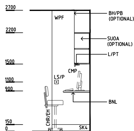
ELEVATION 1
