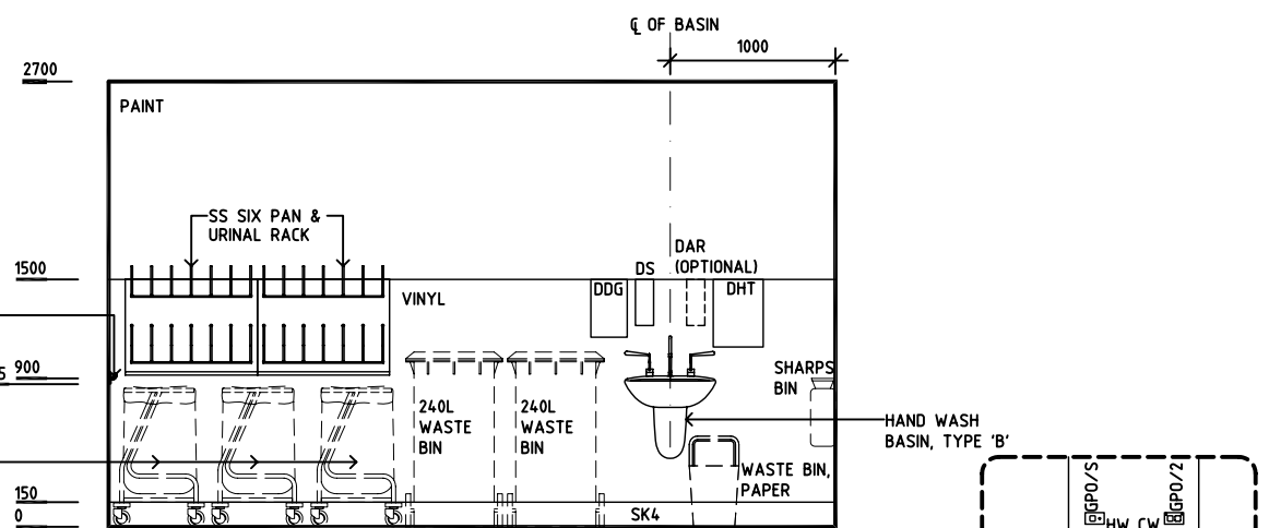
ELEVATION 2
