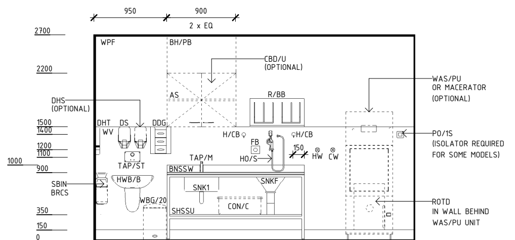
ELEVATION 4
