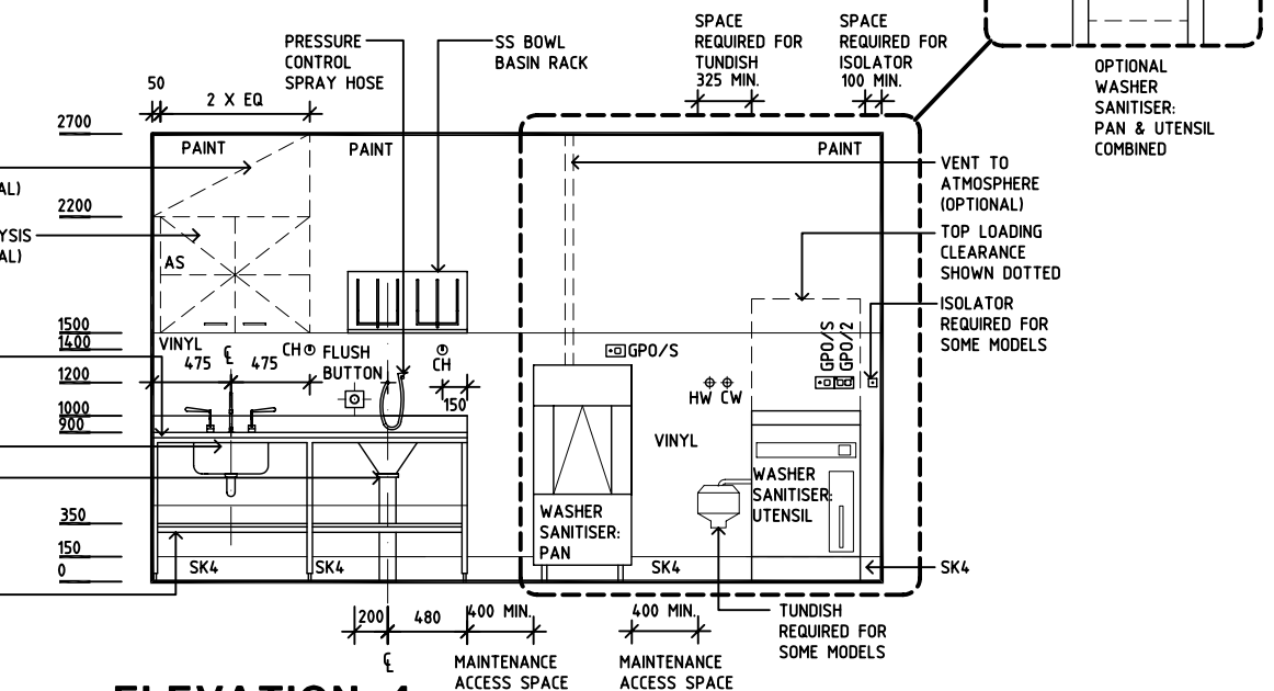
ELEVATION 4
