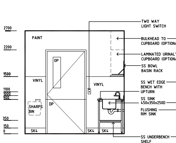
ELEVATION 3
