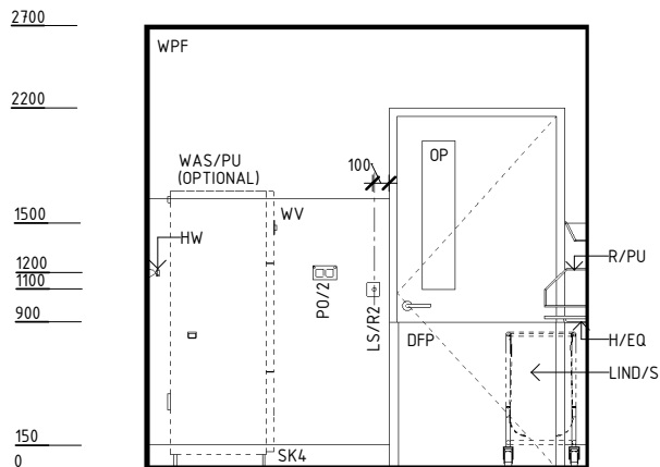
ELEVATION 1
