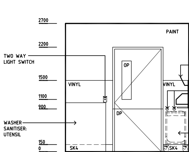
ELEVATION 1
