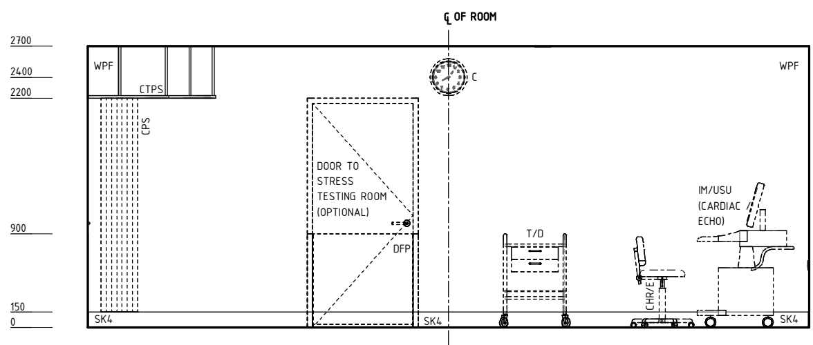
ELEVATION 4
