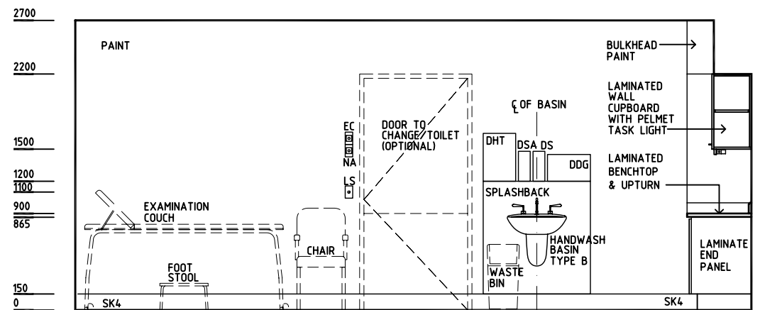
ELEVATION 2
