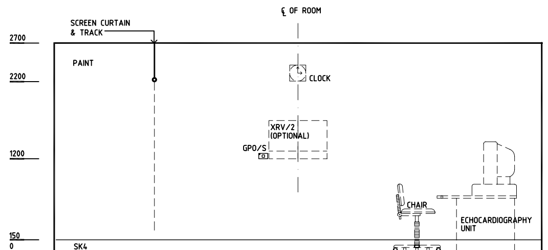
ELEVATION 4
