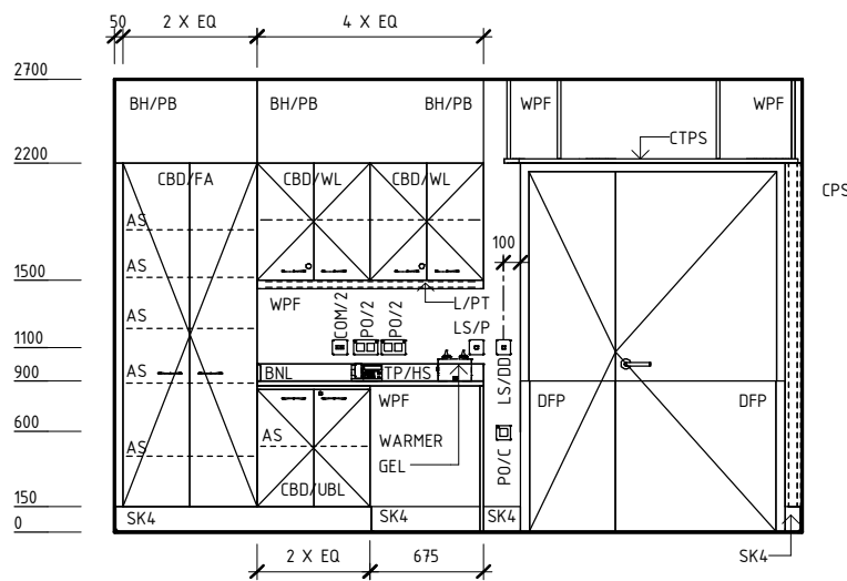
ELEVATION 3
