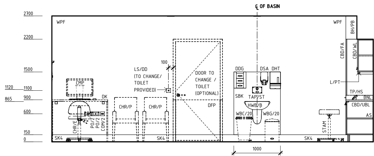
ELEVATION 2
