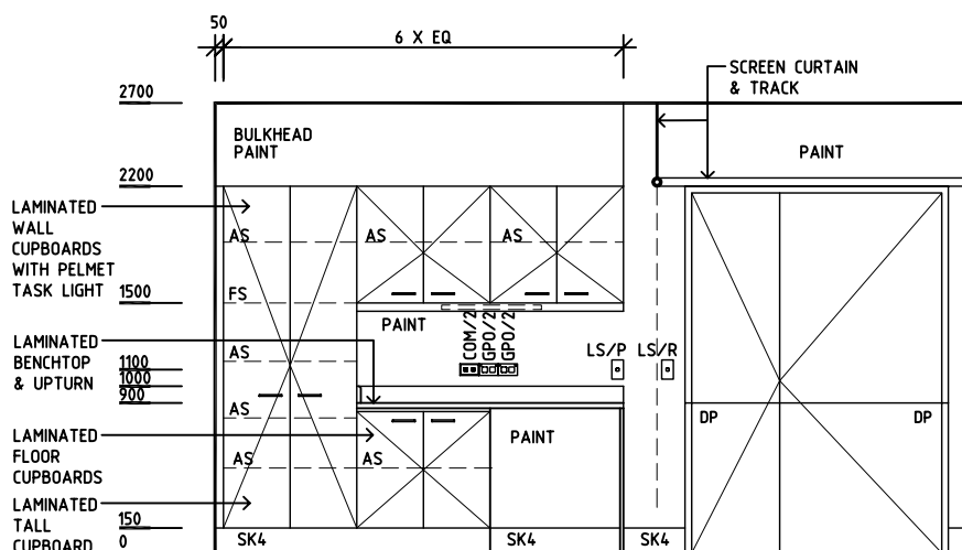
ELEVATION 3
