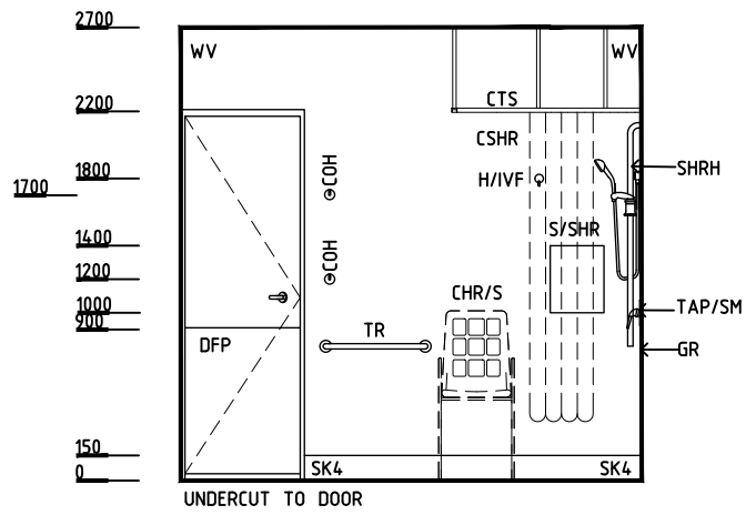
ELEVATION 2
