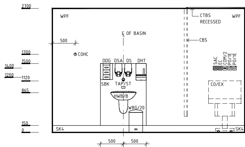
ELEVATION 4
