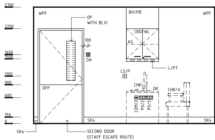
ELEVATION 2
