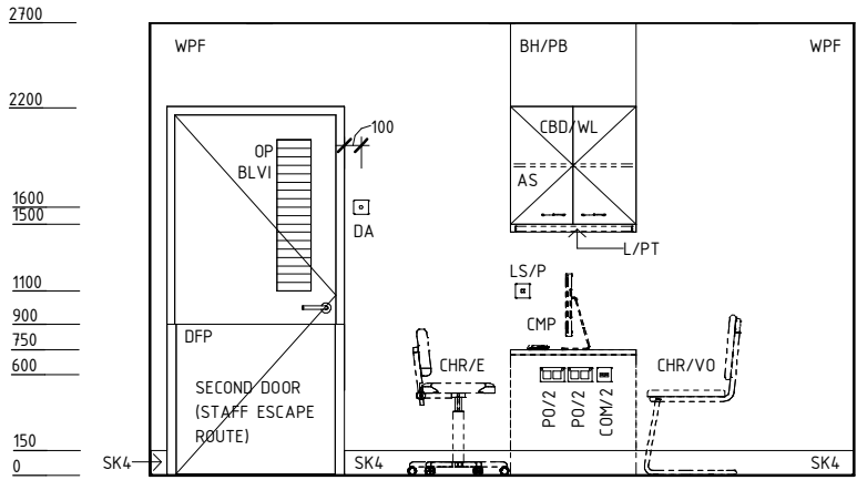
ELEVATION 2
