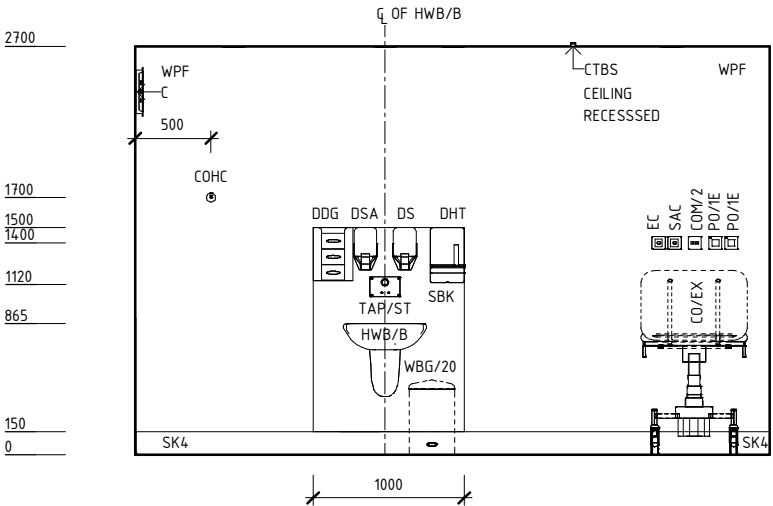
ELEVATION 4
