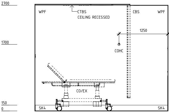
ELEVATION 1
