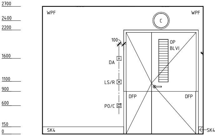
ELEVATION 3
