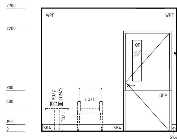
ELEVATION 2
