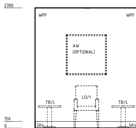
ELEVATION 1
