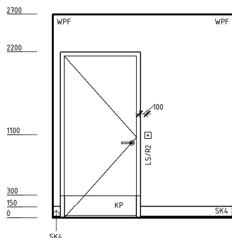
ELEVATION 3
