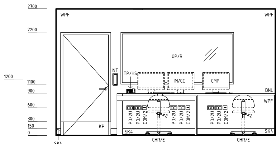
ELEVATION 4
