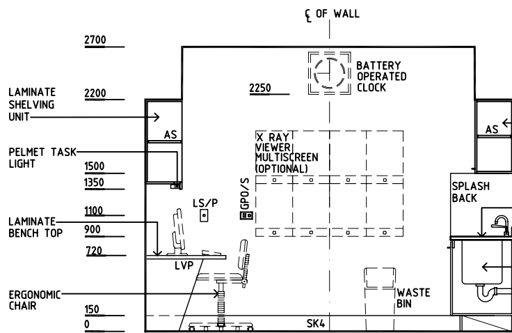
ELEVATION 1
