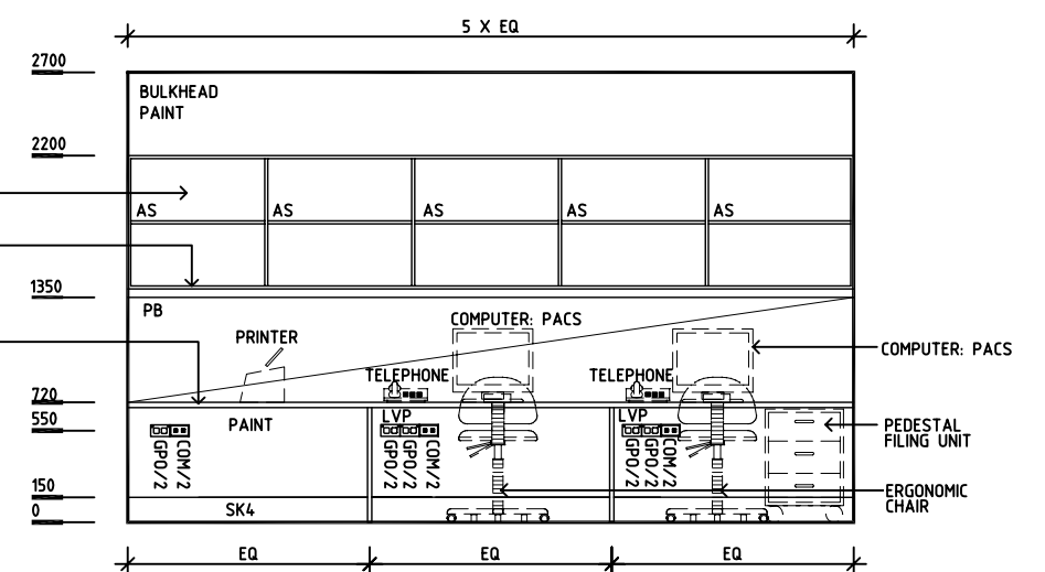
ELEVATION 4
