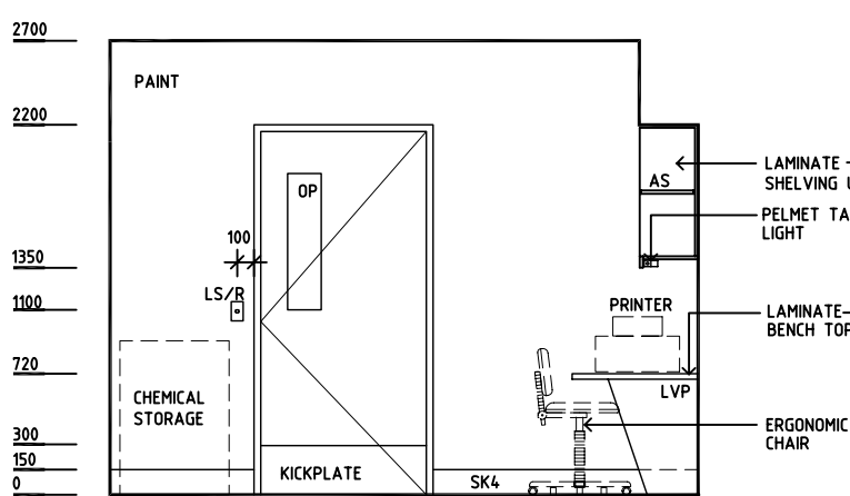
ELEVATION 3
