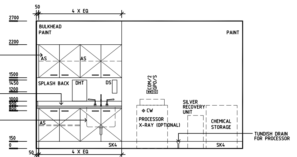
ELEVATION 2
