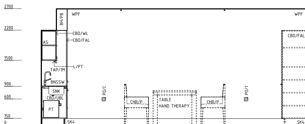
ELEVATION 4
