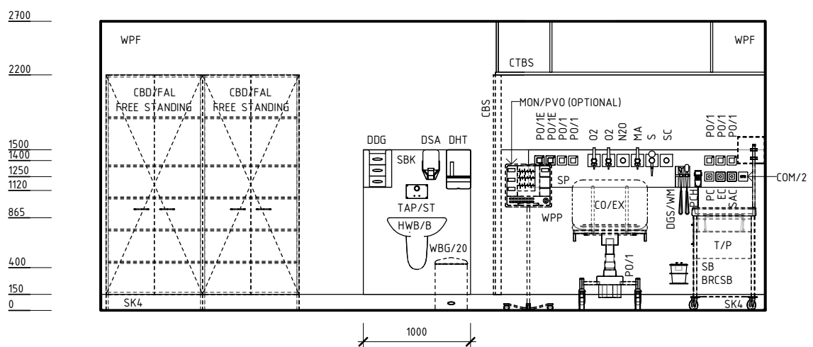
ELEVATION 1
