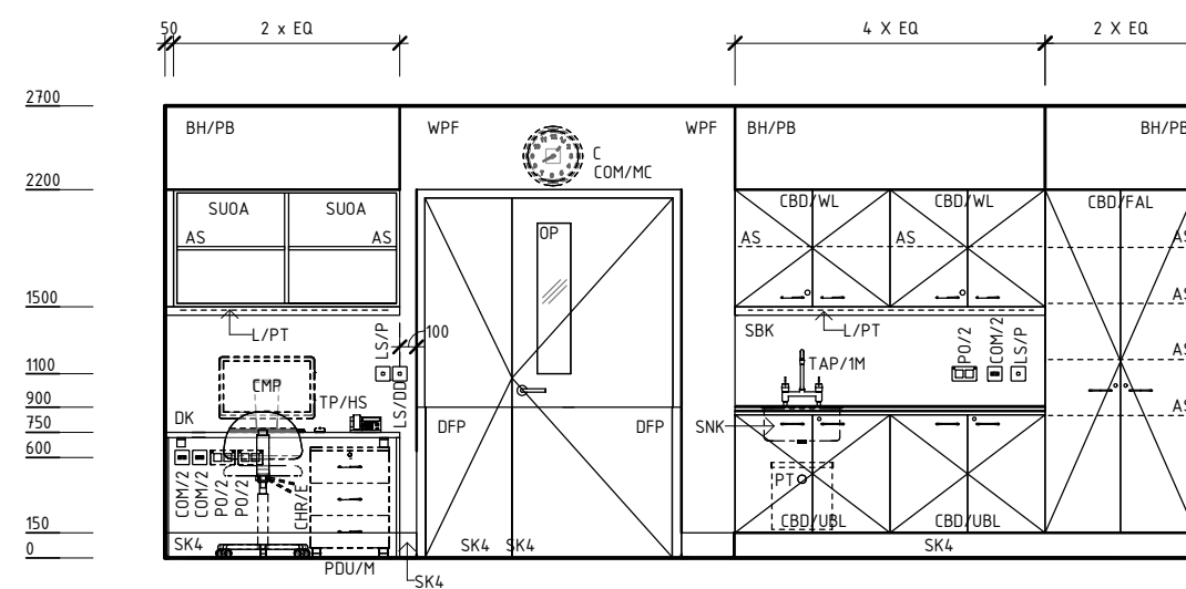
ELEVATION 3
