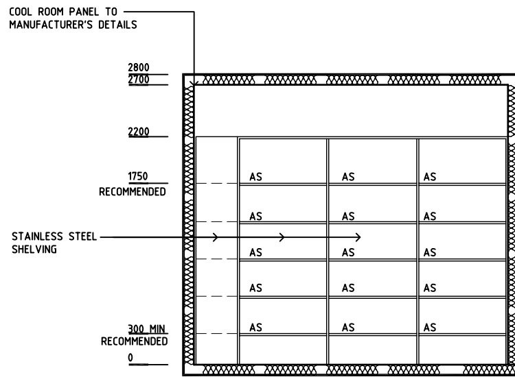
ELEVATION 1
