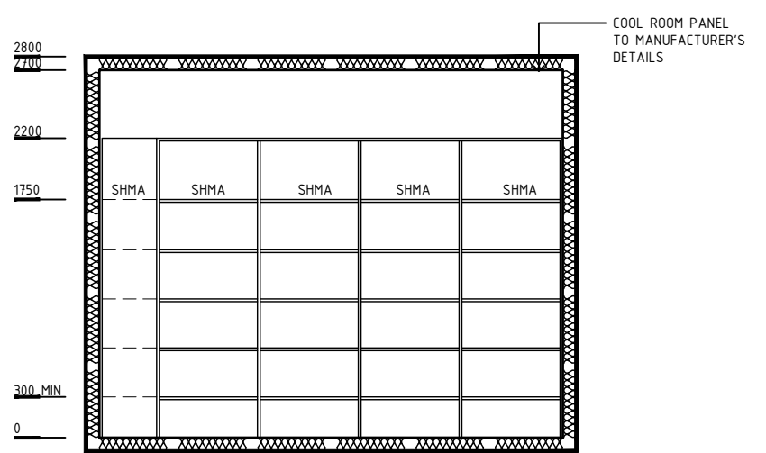
ELEVATION 2
