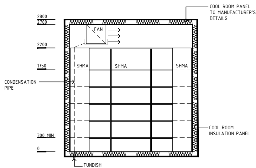
ELEVATION 1
