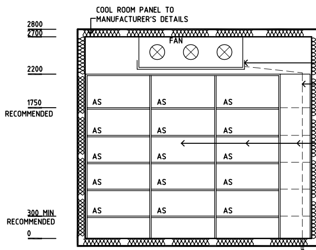
ELEVATION 3
