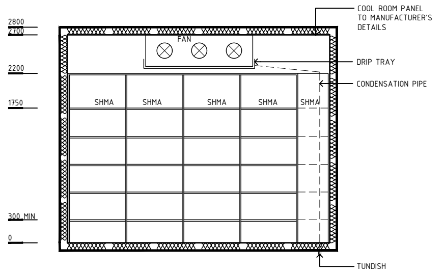
ELEVATION 4
