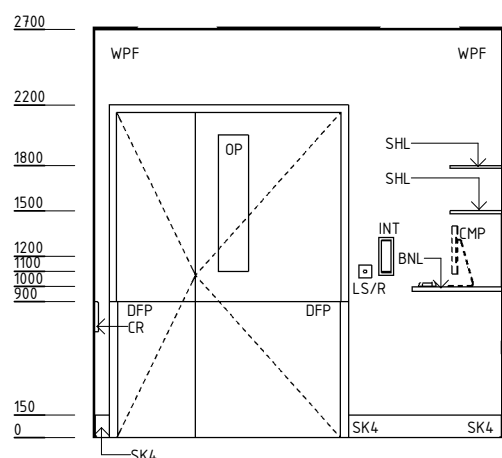
ELEVATION 3
