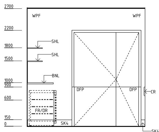
ELEVATION 1
