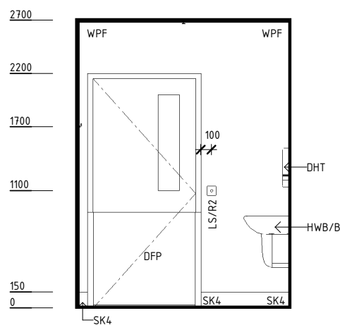
ELEVATION 1
