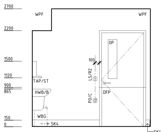
ELEVATION 3
