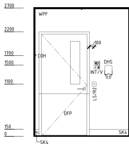
ELEVATION 1
