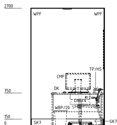
ELEVATION 4
