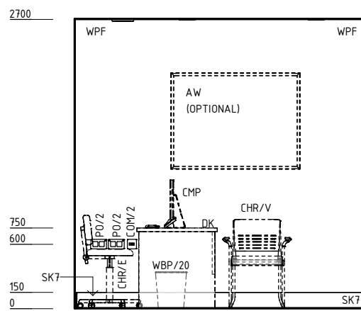
ELEVATION 1
