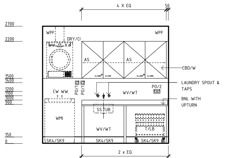
ELEVATION 2
