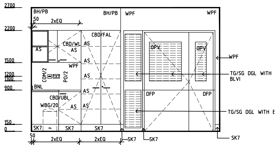
ELEVATION 3
