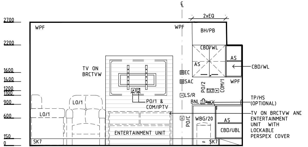
ELEVATION 2
