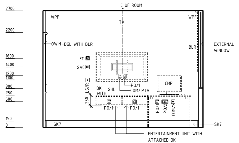
ELEVATION 4
