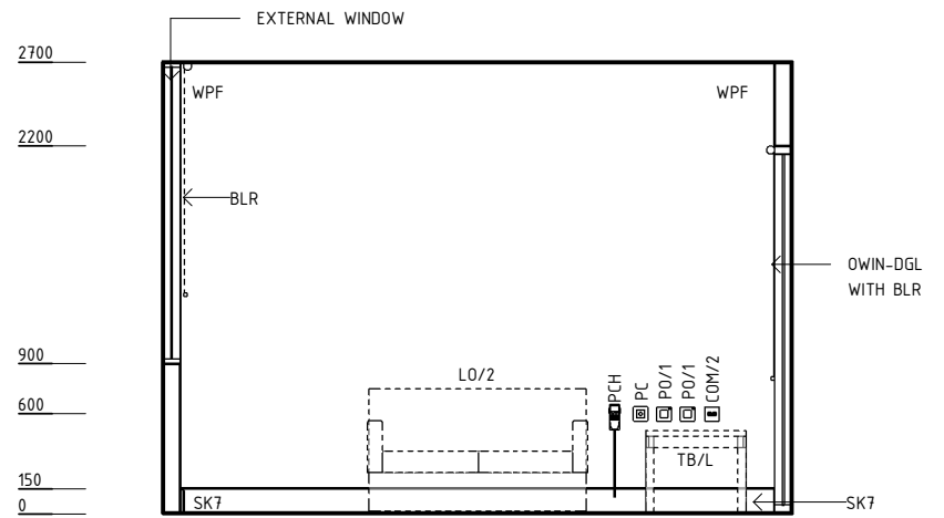
ELEVATION 2
