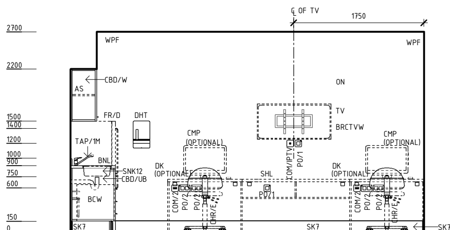
ELEVATION 2
