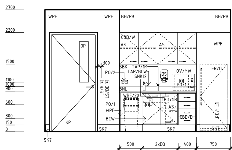
ELEVATION 3
