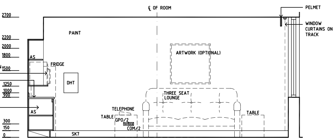
ELEVATION 2
