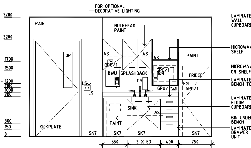
ELEVATION 3
