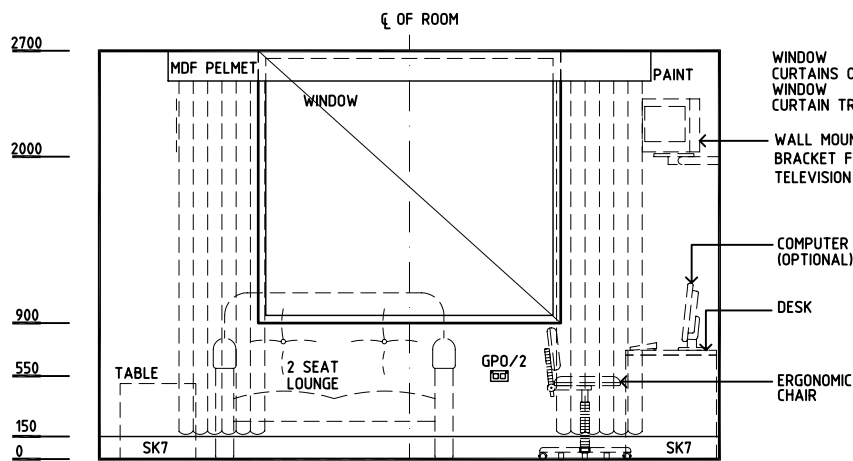
ELEVATION 1
