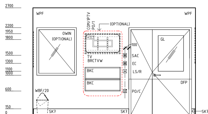
ELEVATION 3
