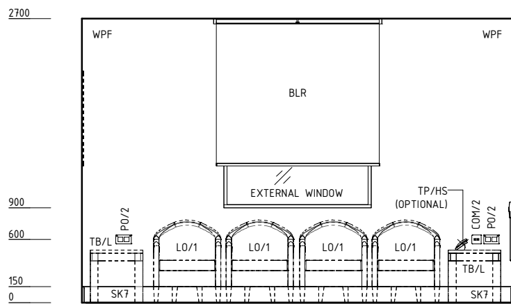
ELEVATION 1
