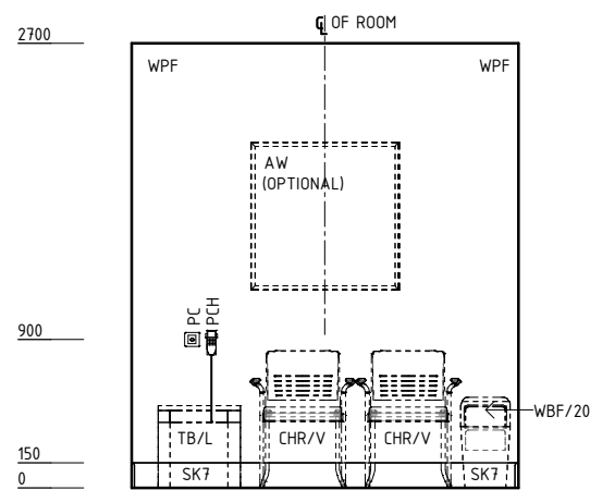
ELEVATION 2
