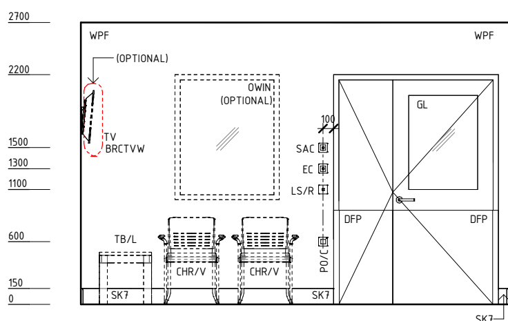
ELEVATION 3
