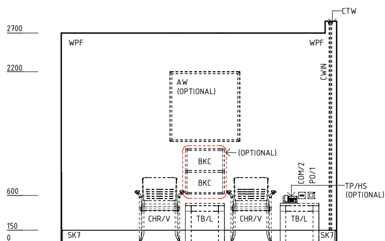
ELEVATION 4
