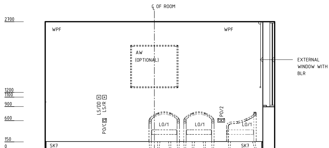
ELEVATION 4
