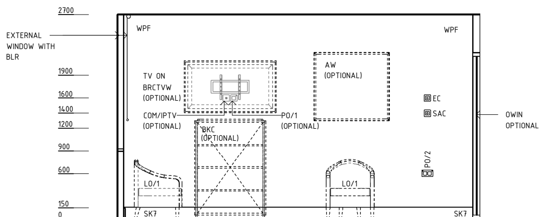
ELEVATION 2
