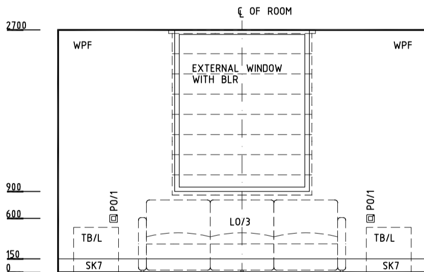
ELEVATION 1
