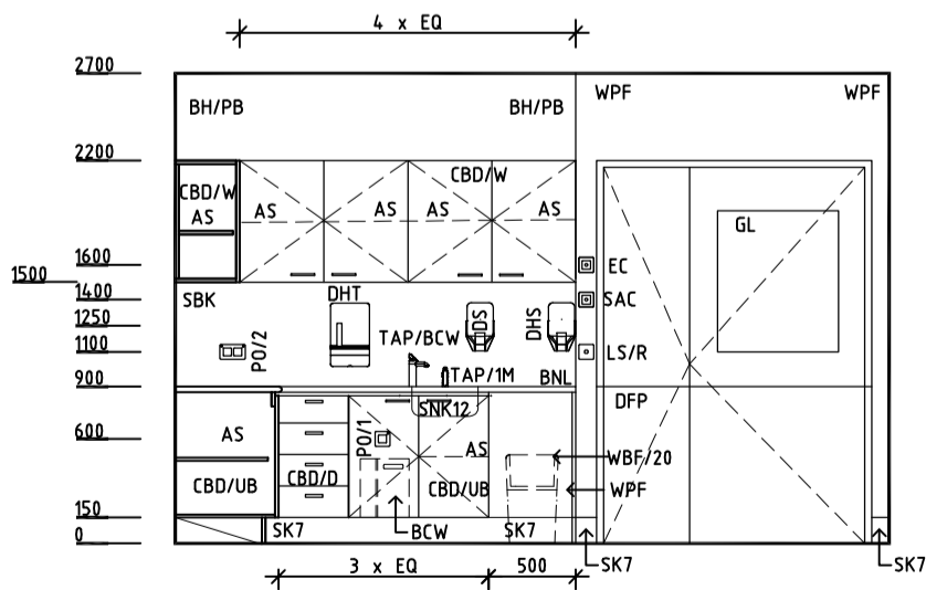
ELEVATION 3
