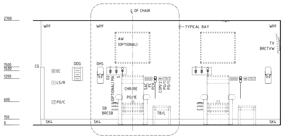
ELEVATION 1
