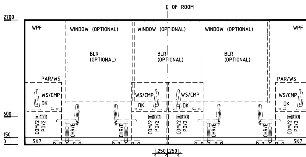
ELEVATION 1
