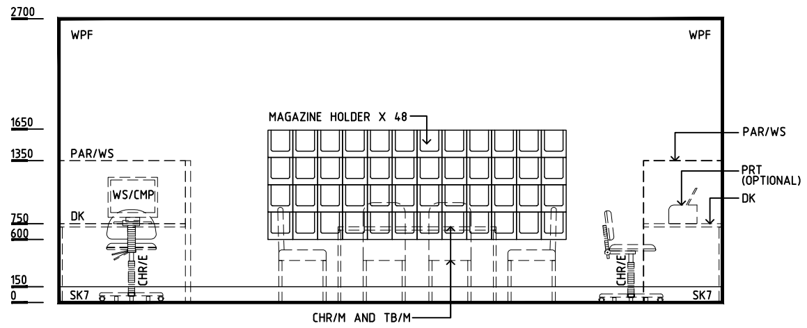
ELEVATION 2
