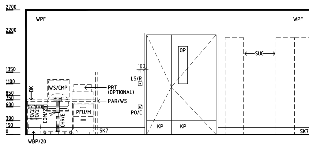
ELEVATION 3
