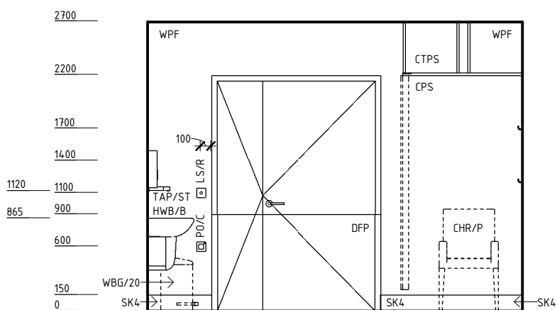
ELEVATION 3
