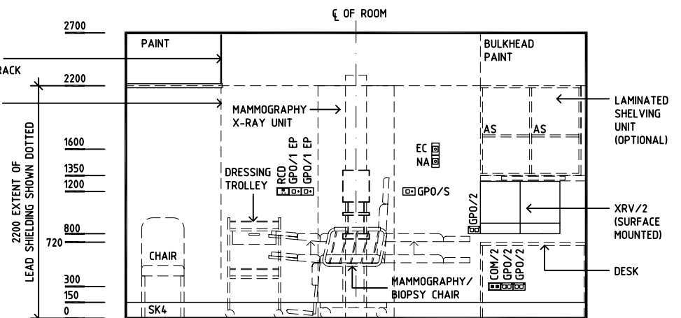
ELEVATION 4
