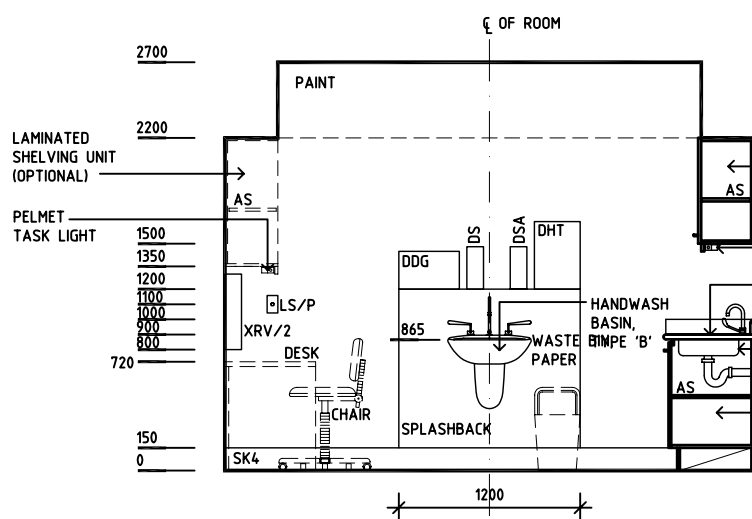
ELEVATION 1
