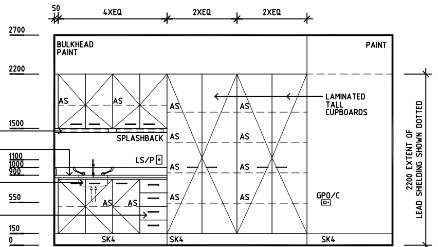
ELEVATION 2
