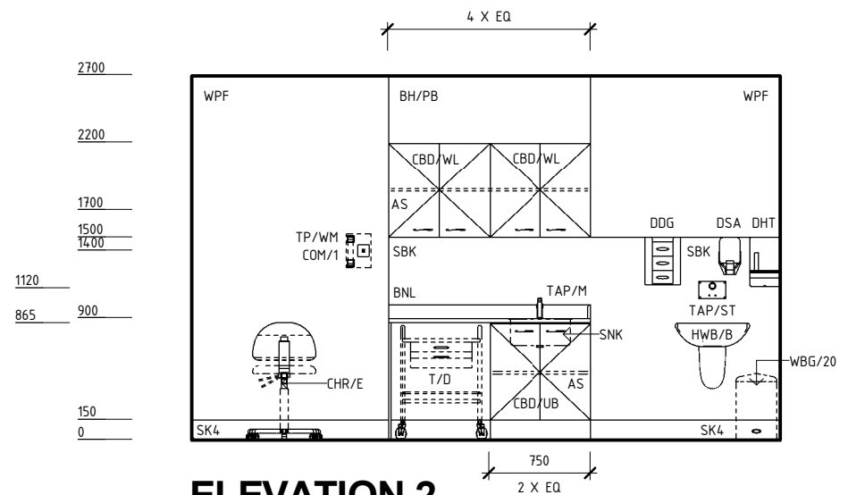
ELEVATION 2
