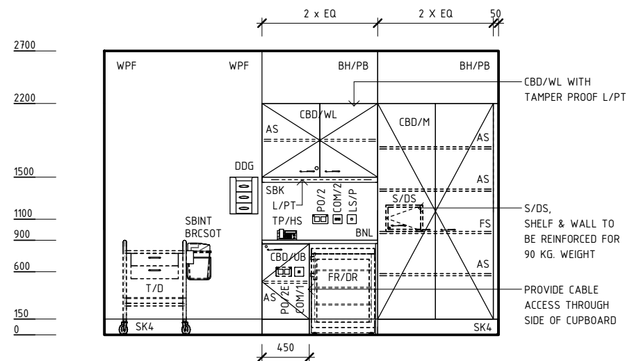
ELEVATION 4
