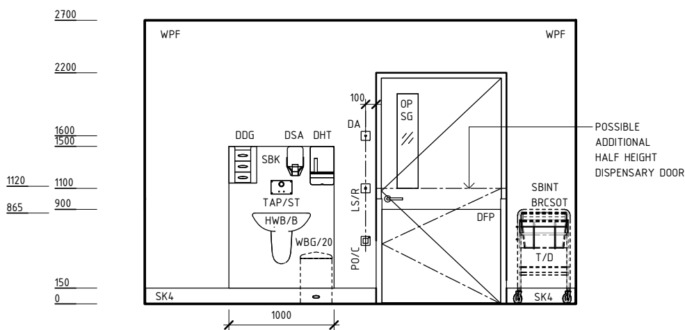
ELEVATION 3
