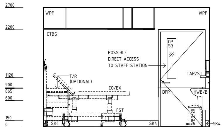
ELEVATION 2
