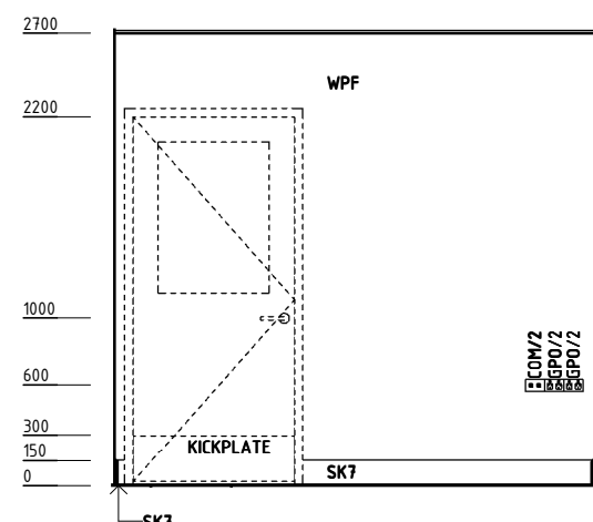
ELEVATION 4
