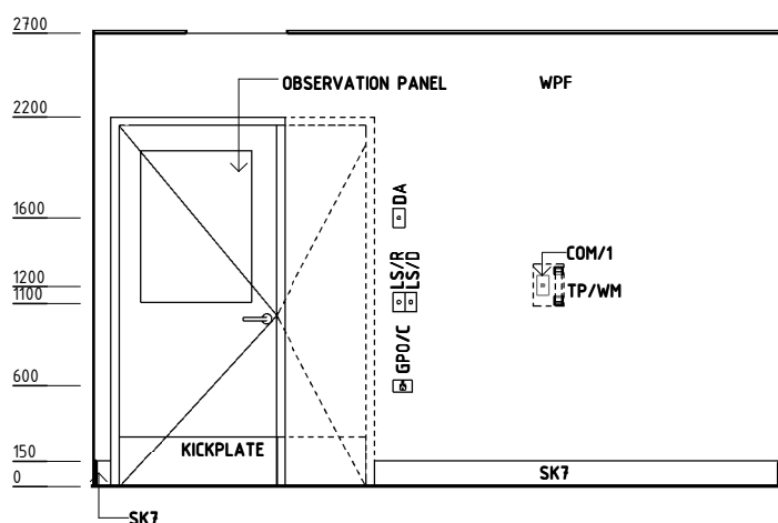
ELEVATION 3
