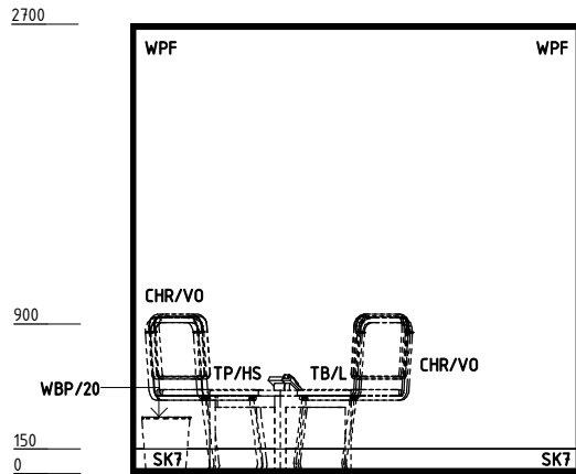
ELEVATION 1
