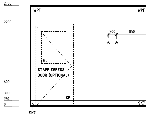
ELEVATION 2
