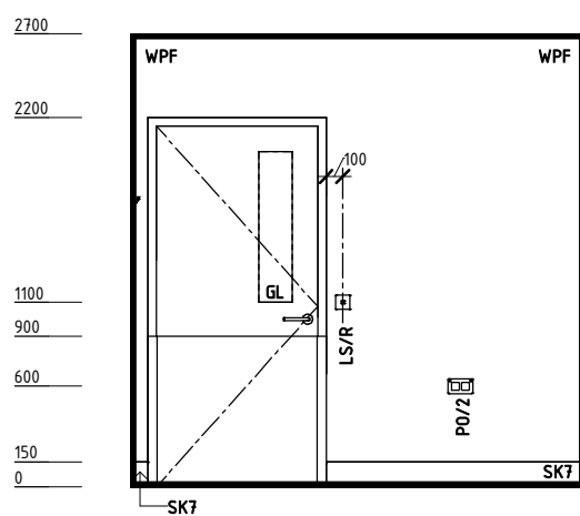
ELEVATION 3
