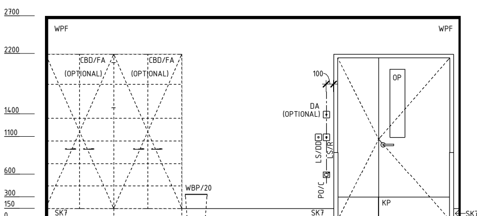
ELEVATION 3
