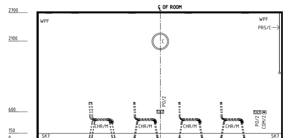
ELEVATION 4
