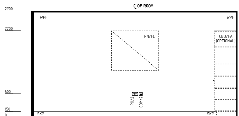
ELEVATION 2
