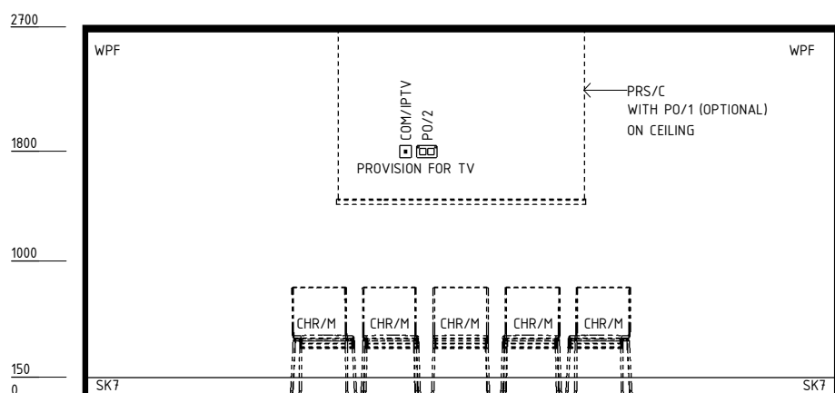
ELEVATION 1
