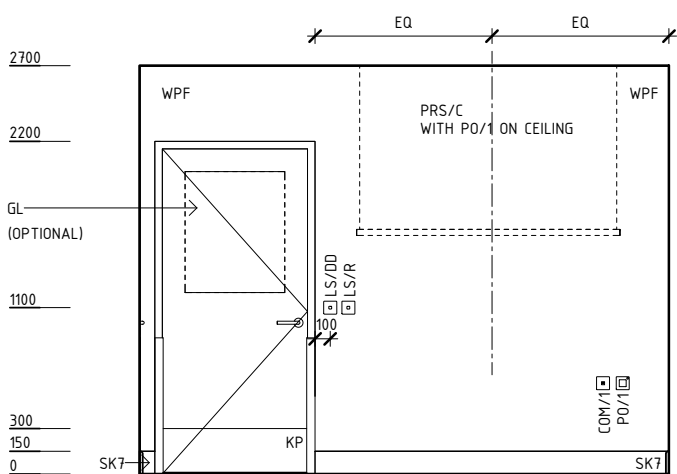
ELEVATION 3
