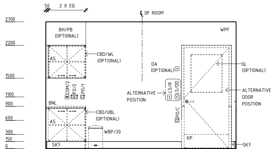
ELEVATION 2
