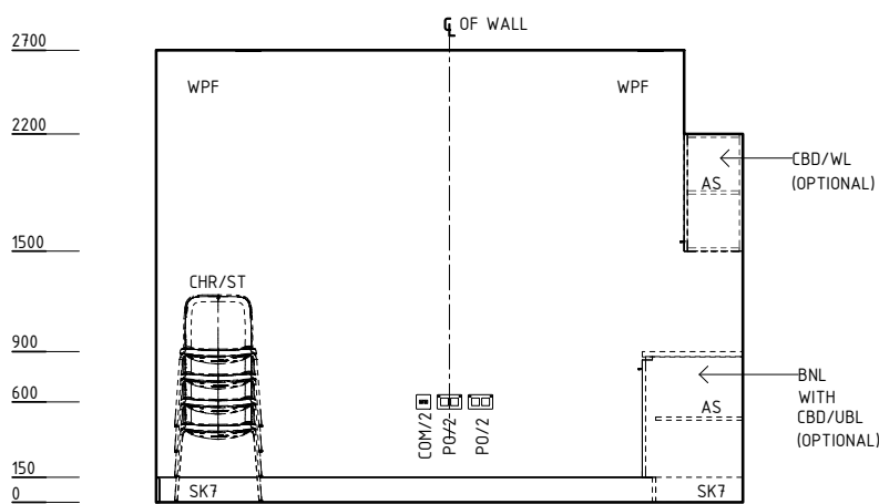
ELEVATION 1
