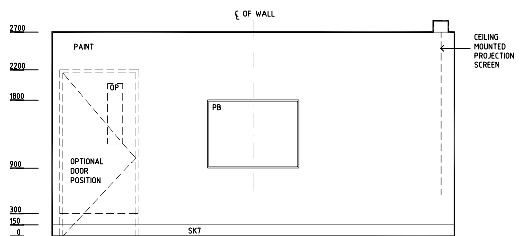
ELEVATION 4
