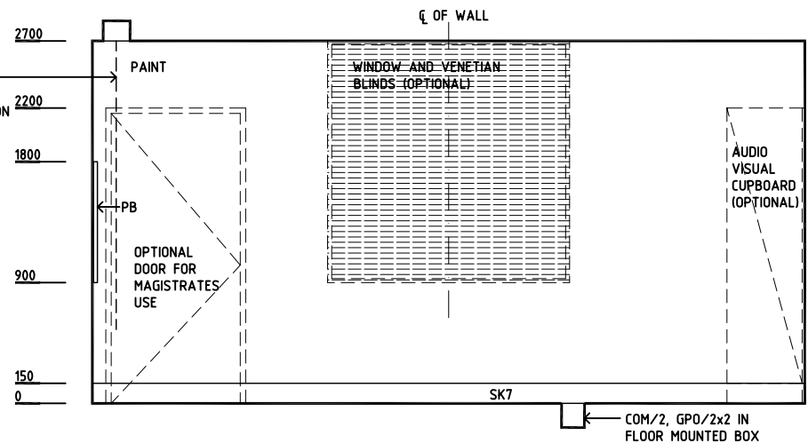
ELEVATION 2
