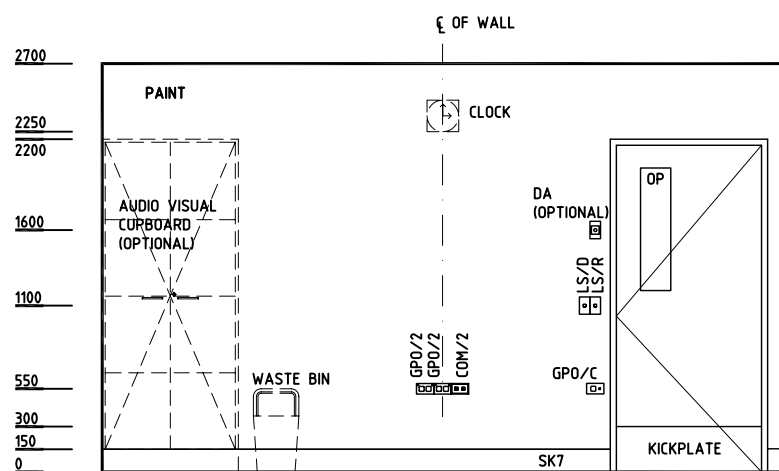
ELEVATION 3
