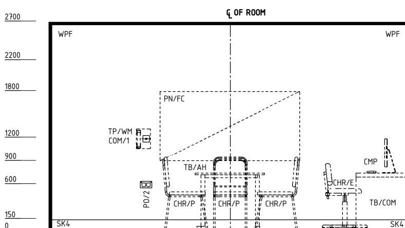
ELEVATION 4
