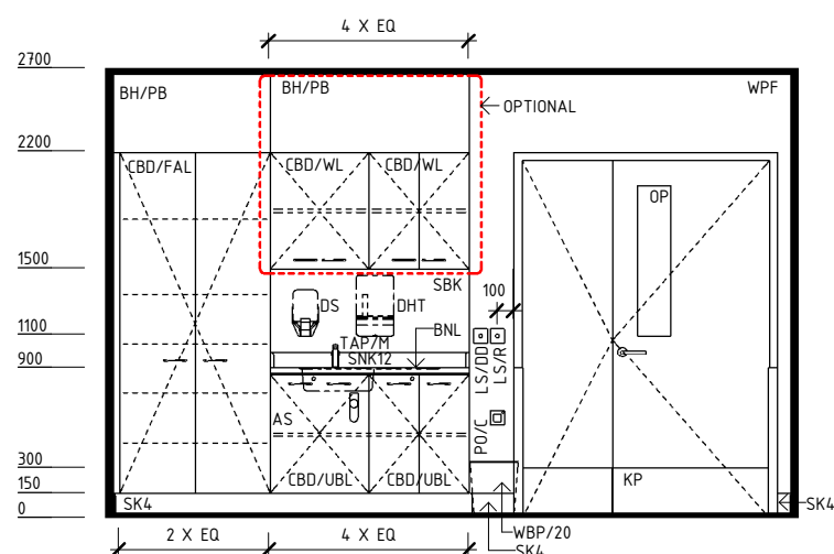
ELEVATION 3
