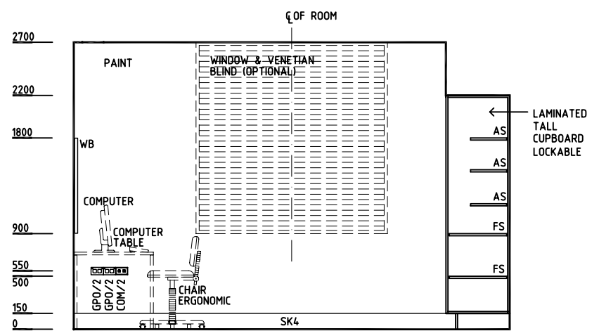
ELEVATION 2
