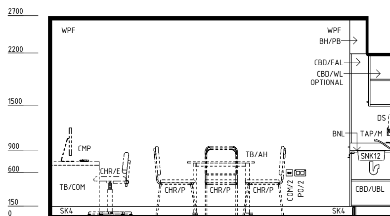
ELEVATION 2
